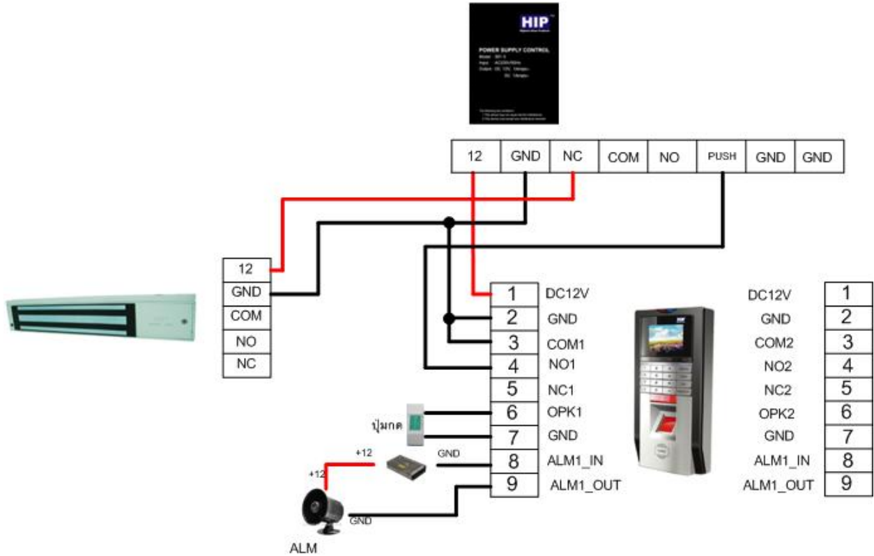
แบบที่ 2 ต่อชุด LOCK ผ่าน POWER SUPPLY
