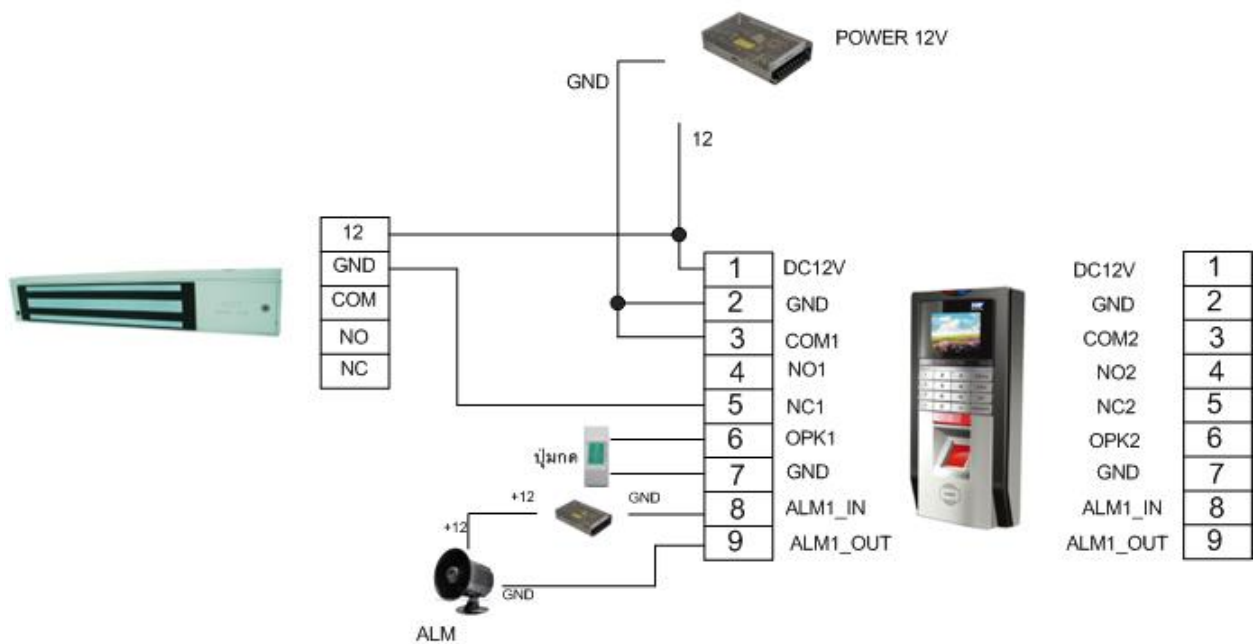
แบบที่1 ต่ออุปกรณ์ LOCK กับเครื่องสแกน
